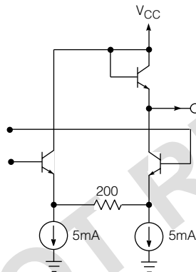
Fig. 8 Pin 16
