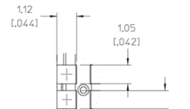
Detail C Scale 10:1 (4) PL.
