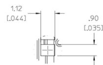
Detail B Scale 10:1 (12) PL.
