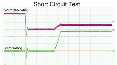
Time-200μs/div
