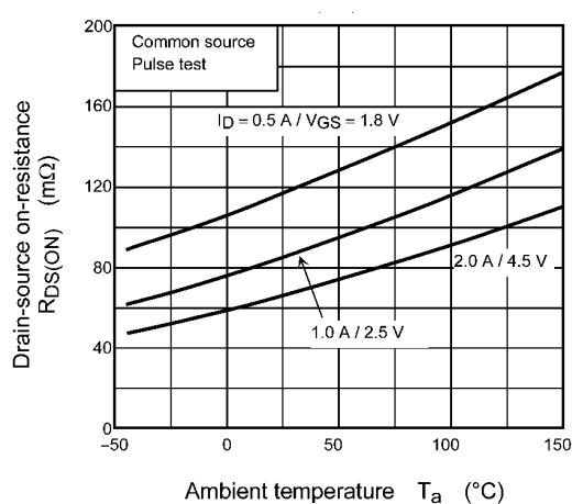
Fig. 7.6 R_{DS(ON)} - T_a
