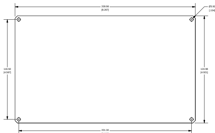
ENCLOSURE LID
