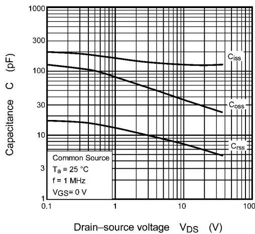
Fig. 7.9 C - V_{DS}
