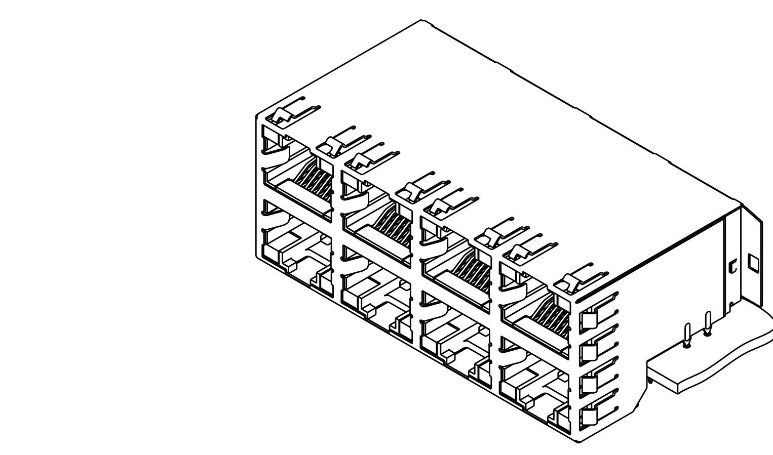
PN 6368062-1, -2, -3, -4, -5, -6, -8 AND 1-6368062-6 SCALE 2:1
