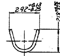
断面“B”-“B”
