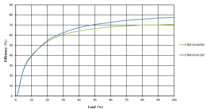
24V Inputs
