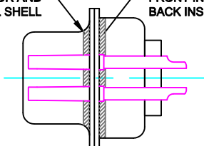
DETAIL A-A
