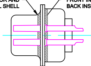
DETAIL A-A
