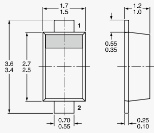
SOD123F
