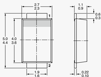
SOD128
