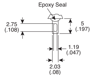
SOLDER LUG
