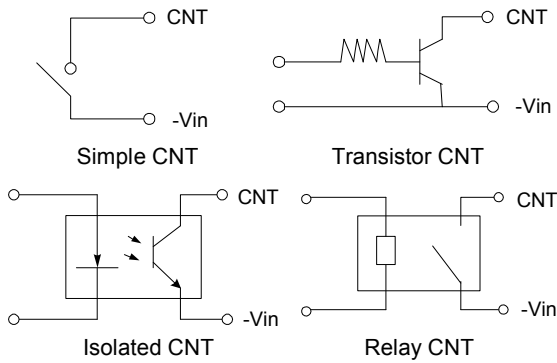
Fig. 71 CNT circuits
