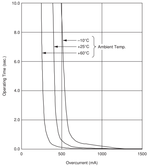
PRG18BC2R2MM1RB
