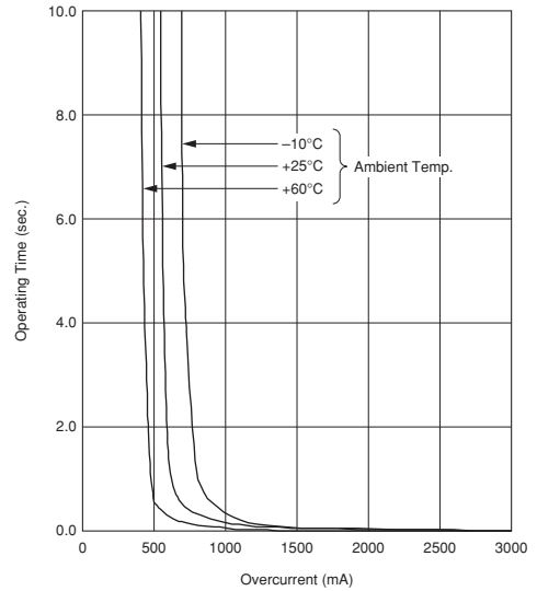
PRG18BC1R0MM1RB
