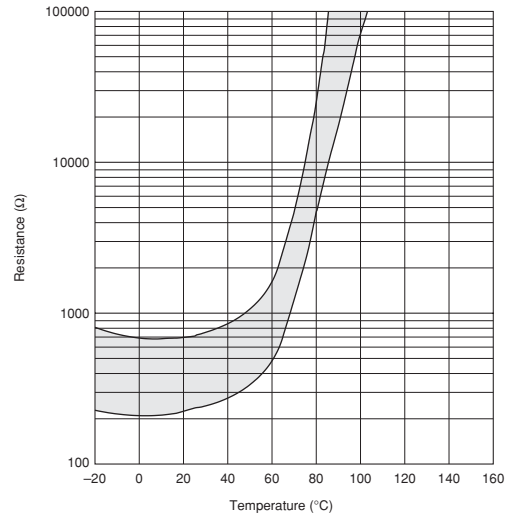
PRF18BF471Q Type
