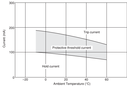
PTGL07AR650H8B52B0
