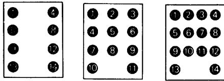
DPDT 3DPT 4DPT
