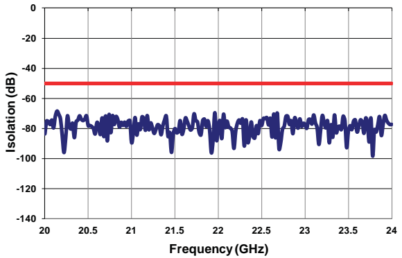
Isolation (20-24 GHz)
