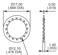
LOCKWASHER
