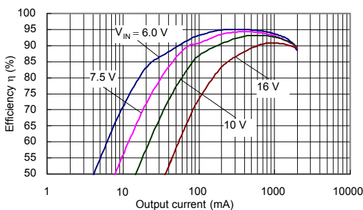
(7) S-8533A50AFT (CPH6302/CPH6402)
