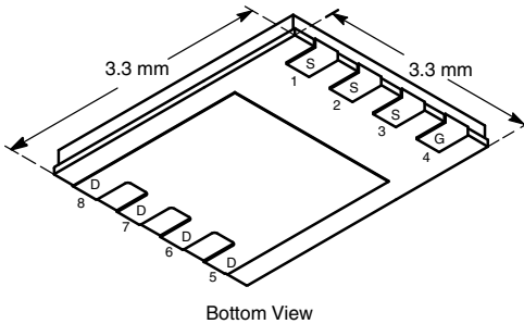
PowerPAK 1212-8
