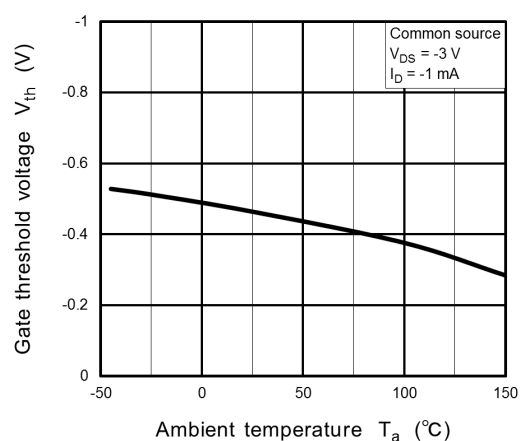
Fig. 7.6 V_{th} - T_a
