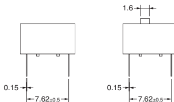
Flat Actuator
