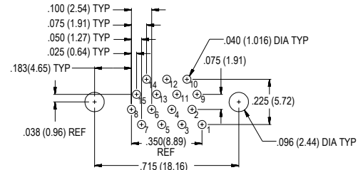
15 PIN MWDM-15PCBS
