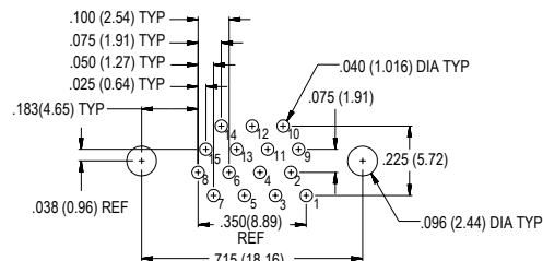
15 PIN MWDM-15PCBS
