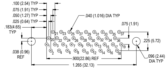
37 Socket MWDM-37SCBS
