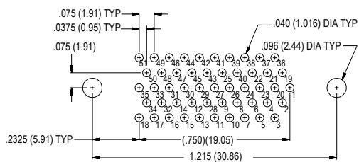
51 PIN MWDM-51PCBS
