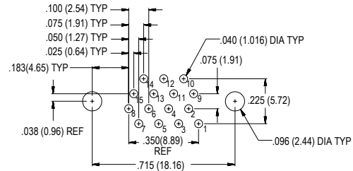
15 PIN MWDM-15PCBS
