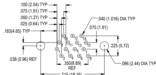
15 Socket MWDM-15SCBS
