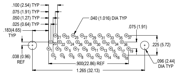
37 Socket MWDM-37SCBS
