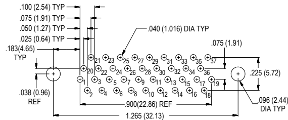
37 Socket MWDM-37SCBS
