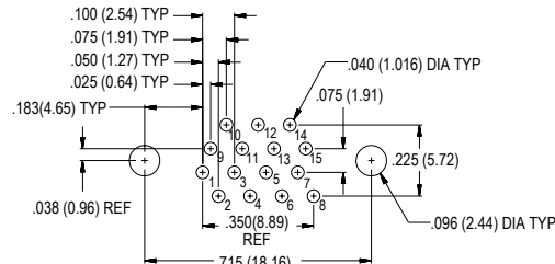
15 Socket MWDM-15SCBS
