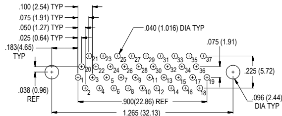
37 Socket MWDM-37SCBS
