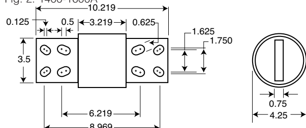
Fig. 2: 1400-1600A
