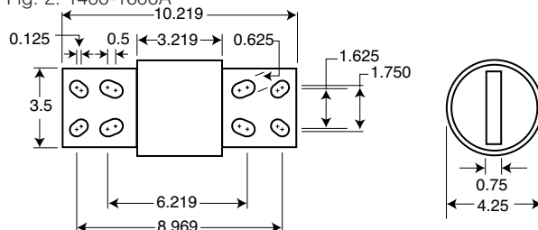
Fig. 2: 1400-1600A
