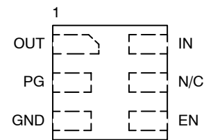
XDFN6
