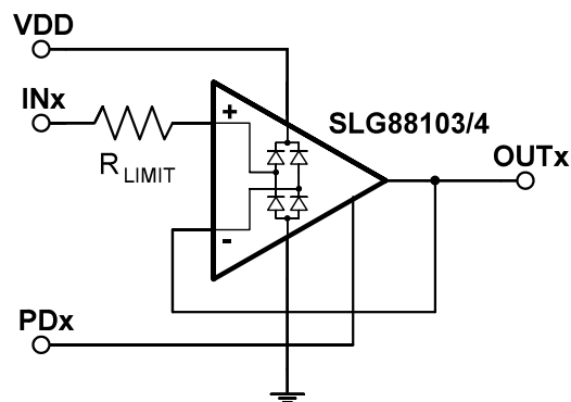
Fig 31. ESD Protection .
