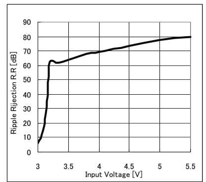
Fig.55 R.R. - VIN
