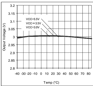
Fig.53 VOUT - Temp
