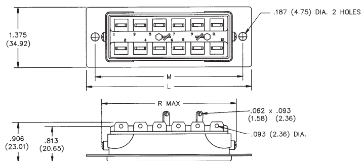
Socket
