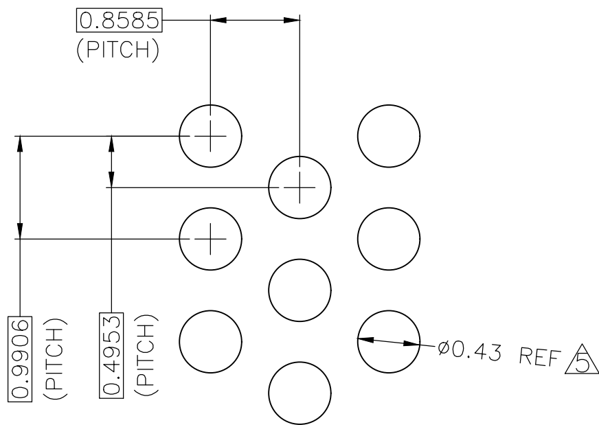
DETAIL M(20:1)
