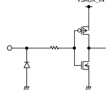
20pin<EC_CLKREQ#>
