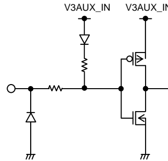
11pin<CPUSB#>
