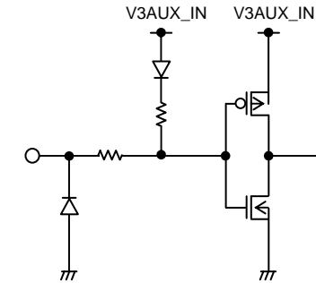
12pin<CPPE#>
