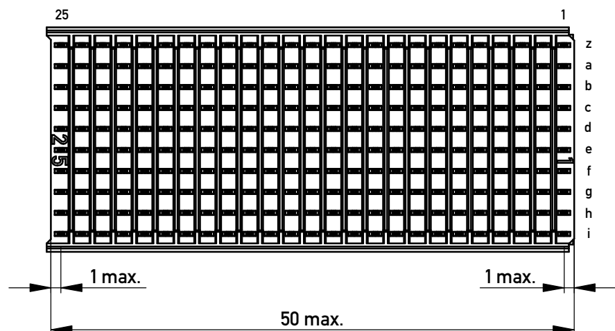
Bestückungsplan / contact layout
