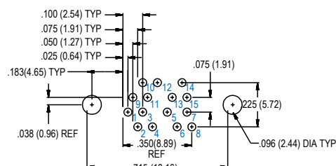
15 SOCKET
