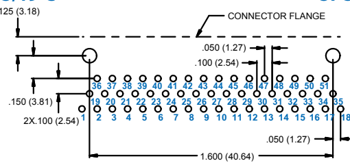
51 SOCKET M83513/20-G
