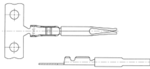
Socket
