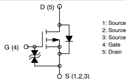
P-CHANNEL MOSFET
