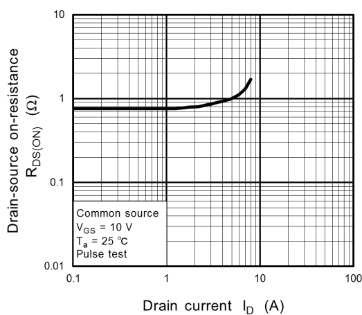
Fig. 8.6 R_{DS(ON)} - I_D
