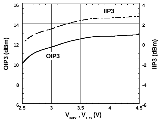
OIP3, IIP3 vs. V_{\text{MIX}}, V_{\text{LO}}
