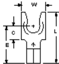
MU10-14FL 1/4 12-10
