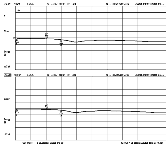
S21, S12
