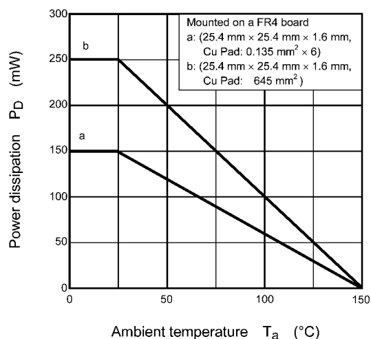
Fig. 7.13 P_D - T_a
