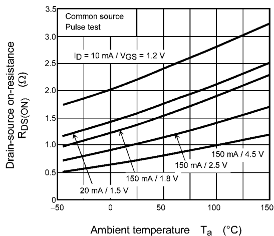
Fig. 7.6 R_{DS(ON)} - T_a
