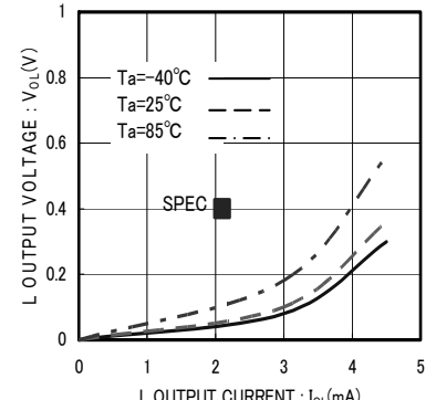
Fig.4 'L' output voltage VOL-IOL(Vcc=3.0V)
