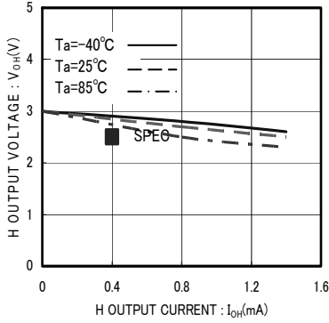
Fig.5 'H' output voltage VOH-IoH(Vcc=3.0V)
