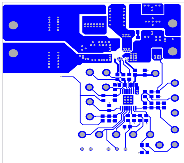
FIGURE 22. TOP LAYER
