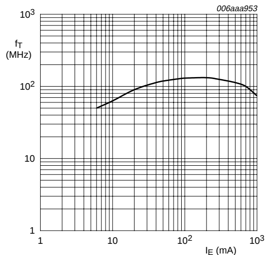
T_{amb} = 25^\circ\text{C} ; V_{CE} = -2\text{ V}
