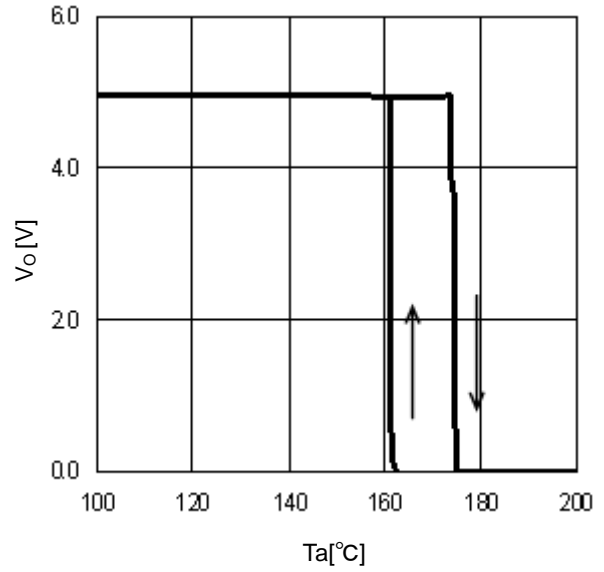
Figure 28. TSD ( I_o=0\text{mA} )
