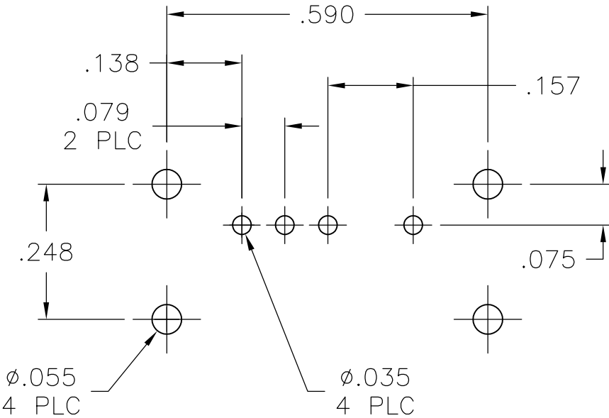
P.C.B. LAYOUT
